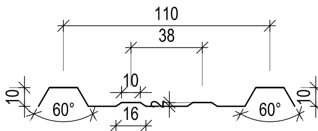
Poprečni presek
