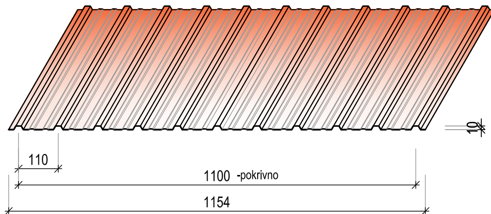
Poprečni presek
