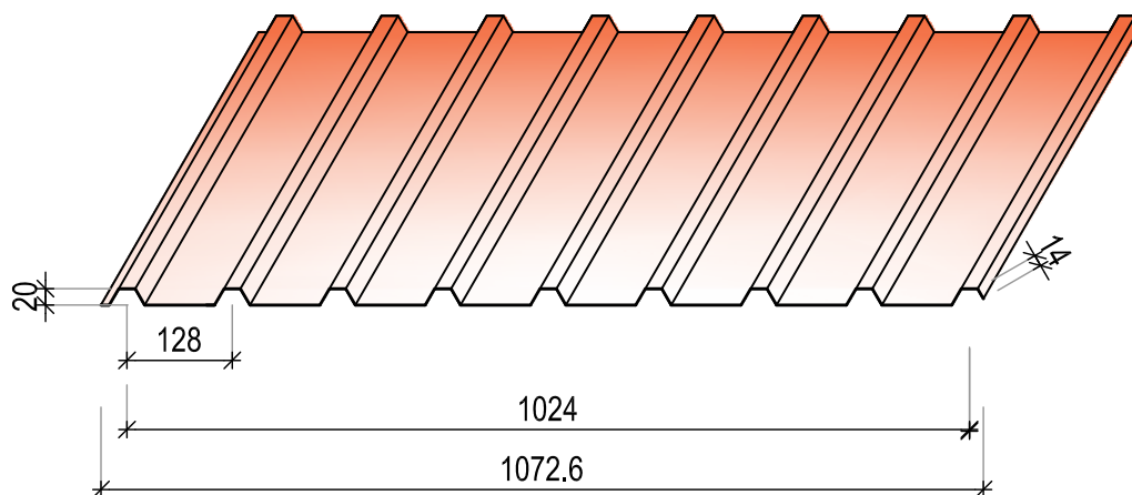
Poprečni presek
