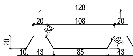
Poprečni presek
